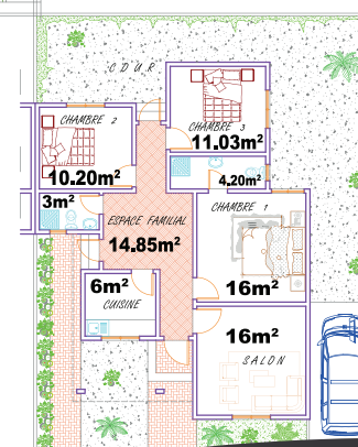
VILLA AMINA REZ-DE-CHAUSSEE 3 chambres + 1 salon Surface habitable : 81,28 m 2 Surface terrain : 200 m 2
