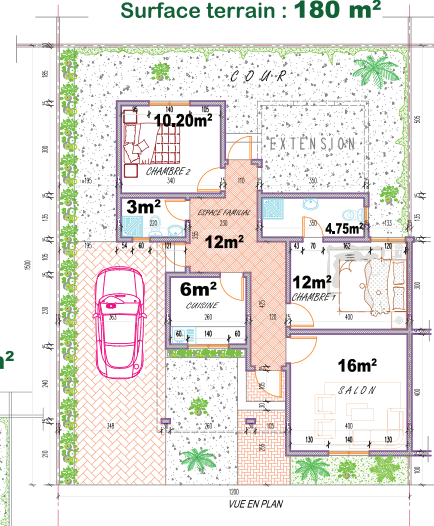
VILLA KHADIJA REZ-DE-CHAUSSEE 2 chambres + 1 Salon Surface habitable : 63,95 m 2 Surface terrain : 180 m 2
